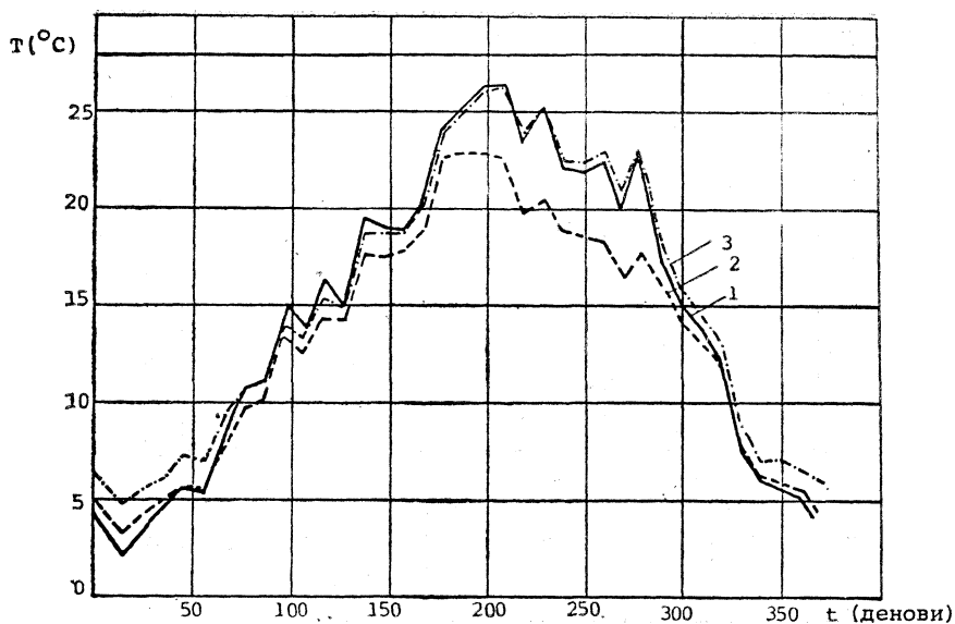
Сл. 6 — Годишна промена на температурата на водата на р. Вардар: 1) пред вливот на р. Црна, 2) после вливот на р. Црна во амбиентни услови, 3) после вливот на р. Црна при ладење на ХЕ со моќност од 1246 MWe.
