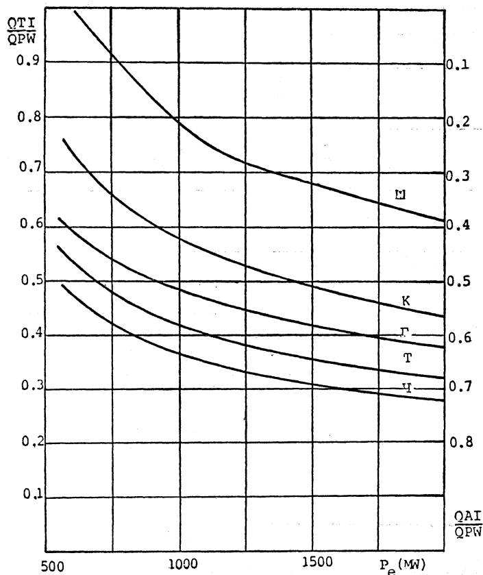
Сл. 8 — Релативен однос на одведената топлина преку турбинскиот истек ( Q_{TI} ), односно преку површината на езерото ( Q_{AI} ) во однос на вкупната отпадна топлина ( Q_{PW} ) за акумулациите: Ш — Шпиље, К — Козјак, Г — Галиште, Т — Тиквеш, Ч — Чебреш.
