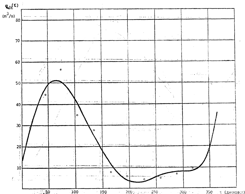
Сл. 3 — Прогнозиран дотек во акумулацијата „Чебрен“
