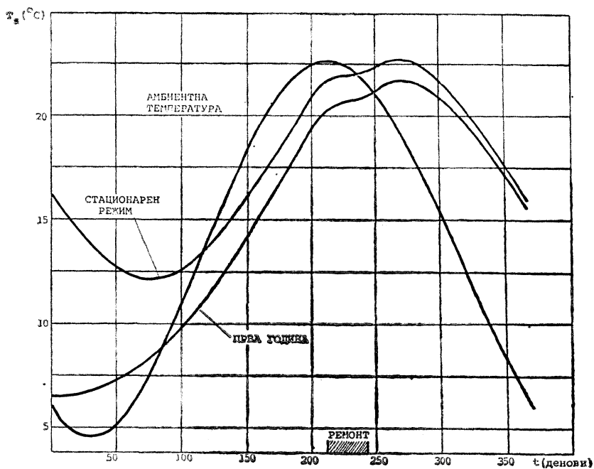
Сл. 5 — Амбиентна и пореметена температура на површината на водата во акумулацијата „Чебрeн“ со лоцирана нуклеарна електрана од 2 \times 632 MWe
