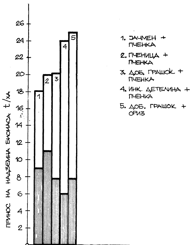
Сл. 8 — Резултати од полски опити со одгледување на две култури годишно (1976/77 и 1977/78)
