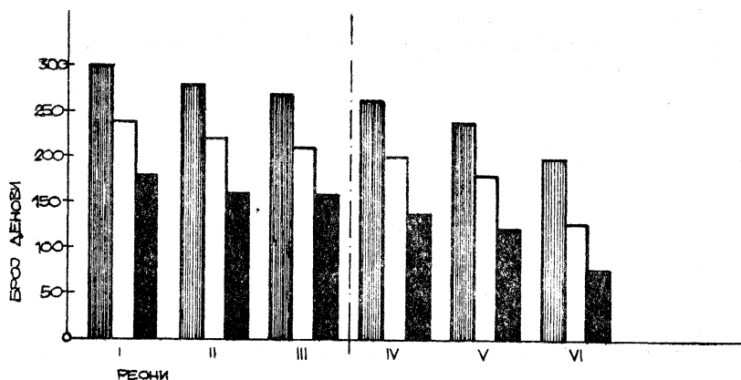
Сл. 4 — Број денови со просечни среднодневни температури на воздухот = 5°C, 10°C и 15°C
