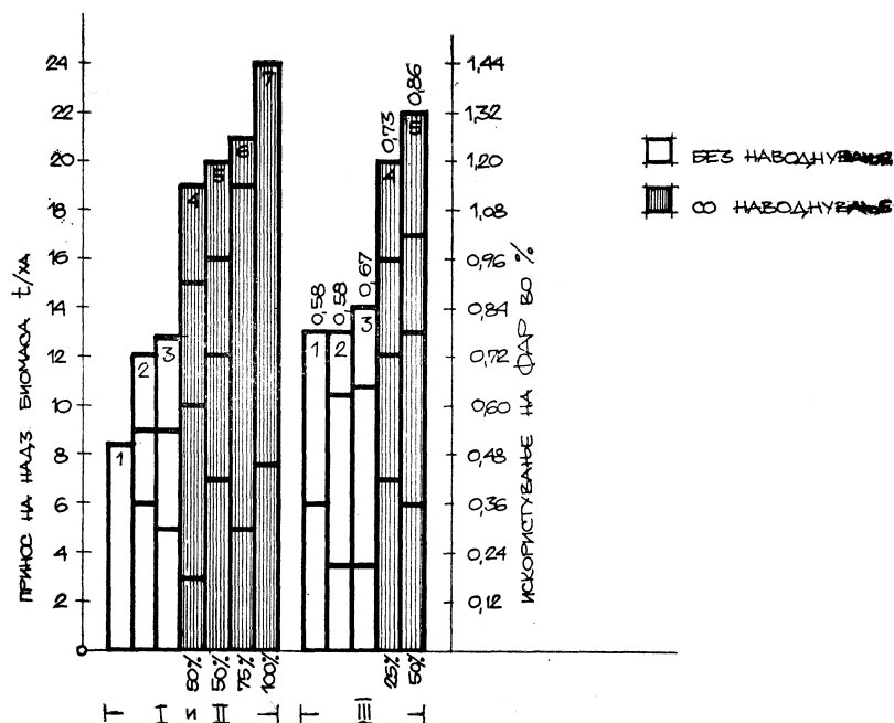
Сл. 9 — Вкупни приноси на надземна биомаса t/ha, % на искористување на ФАР и искористување на ТВС кај некои претпоставени примери на сеидбена структура
