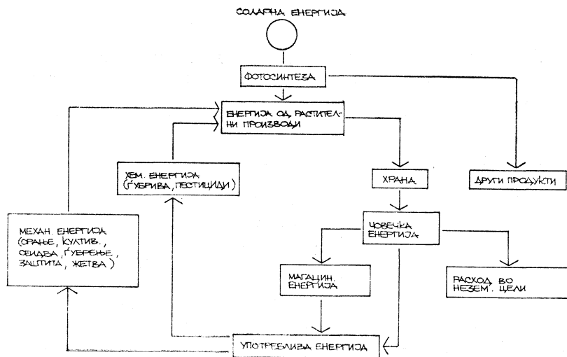
Сл. 2 — Енергетски циклус на растителното производство (Adler et al. 1976)
