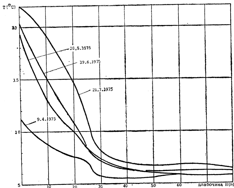
Сл. 1 — Годишна промена на амбиентната температура на водата во Шпиље
