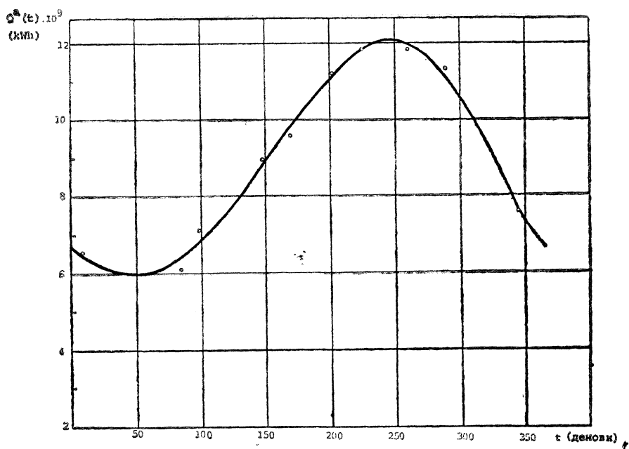
Сл. 4 — Прогнозирана временска зависност на амбиентната топлотна состојба на водата во акумулацијата „Чебрeн“
