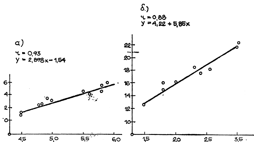
Сл. 6 — Зависност на приносот на надз. биомаса од ФСП а) пченица б) пченка
