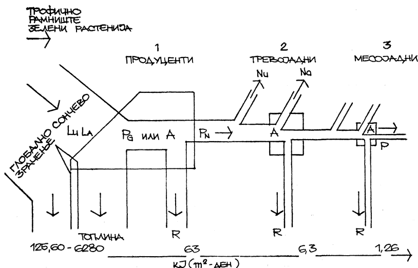
Сл. 1 — Упростен дијаграм на протокот на енергијата низ три (1, 2 и 3) трофични рамништа (1971)
