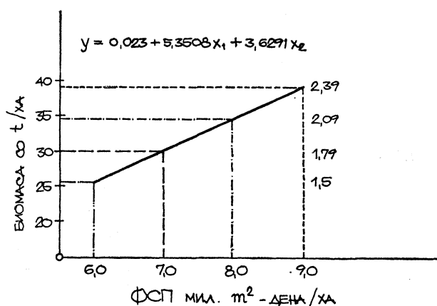
Сл. 7 — Претпоставена потенцијална продуктивност t/ha биомаса
