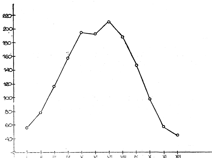
Сл. 3 — Средни месечни суми на глобално сончево зрачење (kWh/m²) (според Поповиќ et al. — 1978)
