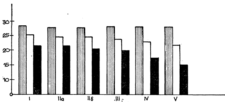
Сл. 5 — Просечен прилив на ФАР во илјада GJ/ha годишно, за период од \geq 5^{\circ}\text{C} и 10^{\circ}\text{C} (според податоци од Поповић et al. 1978)
