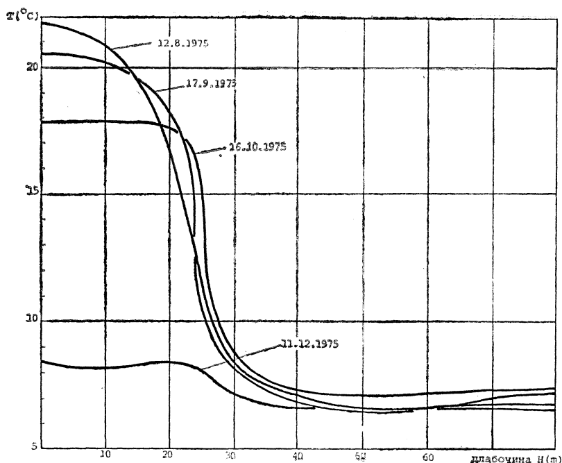
Сл. 2 — Годишна промена на амбиентната температура на водата во Шпиље
