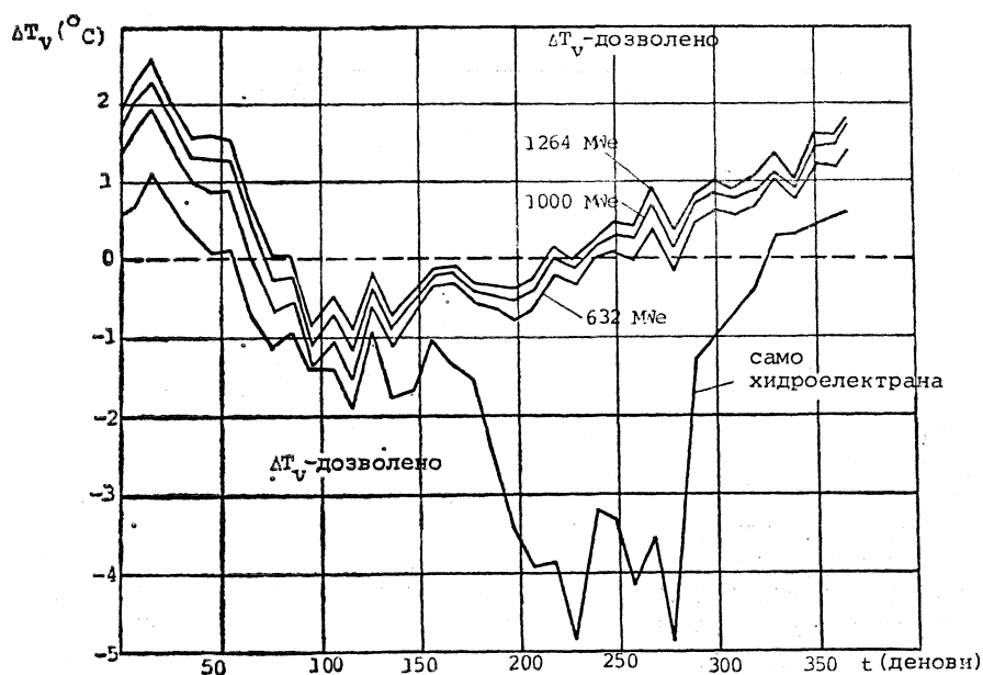
Сл. 7 — Годишна промена на прирастот на температурата на водата на р. Вардар за различна моќност на лоцирани „ХЕ“ ладени со водите на акумулацијата „Тиквеш“
